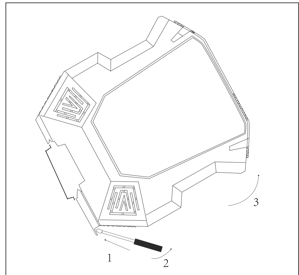
拆卸图
