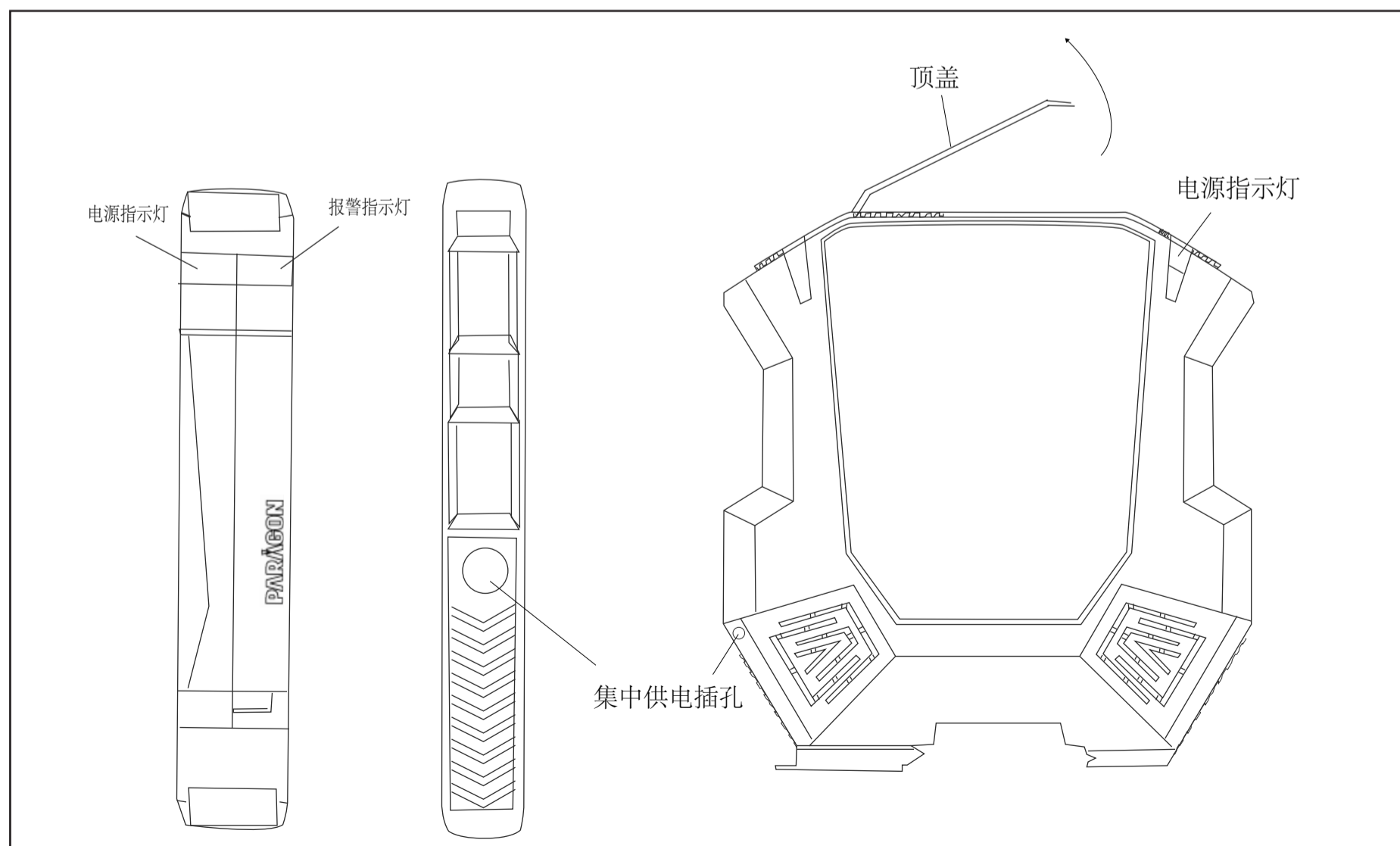
结构图
