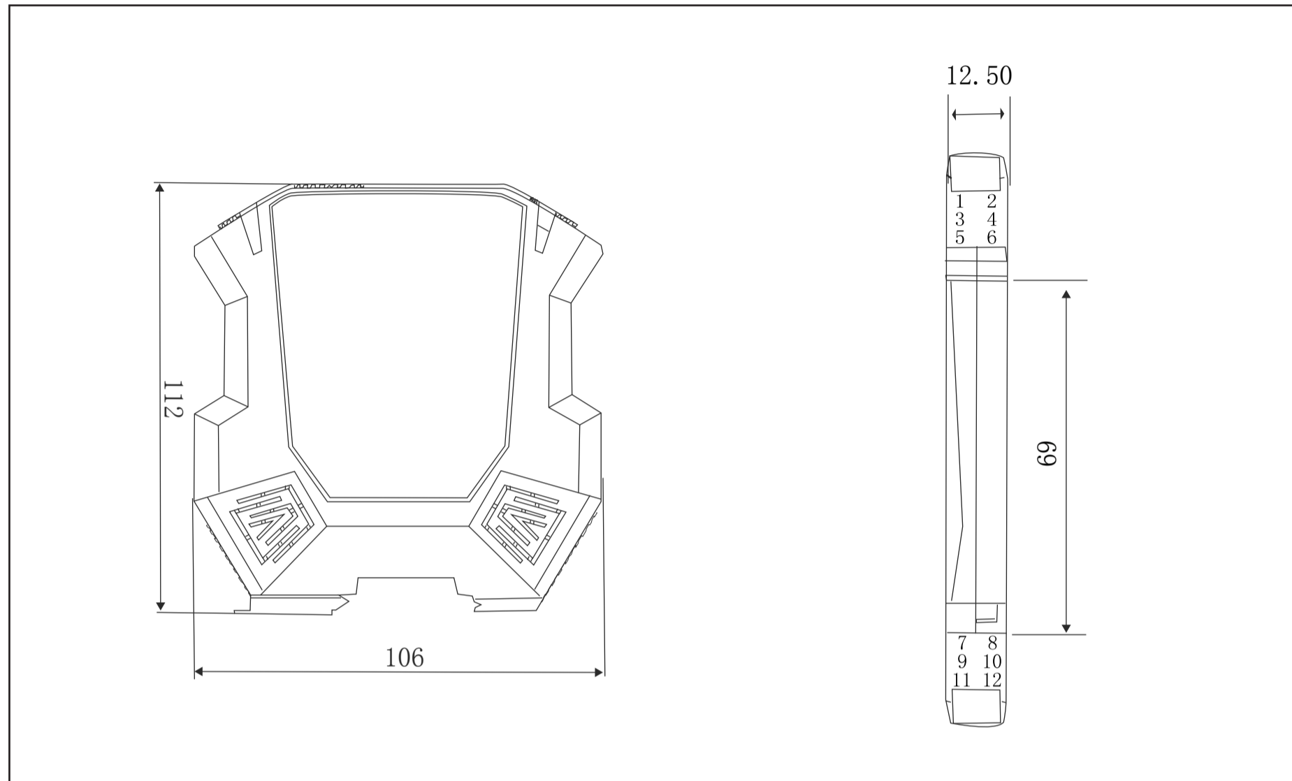
尺寸图
