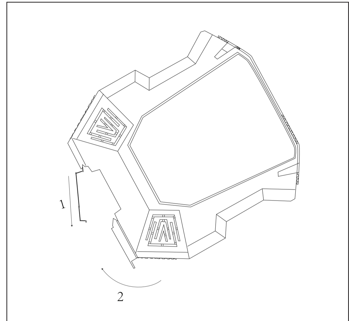
安装图
